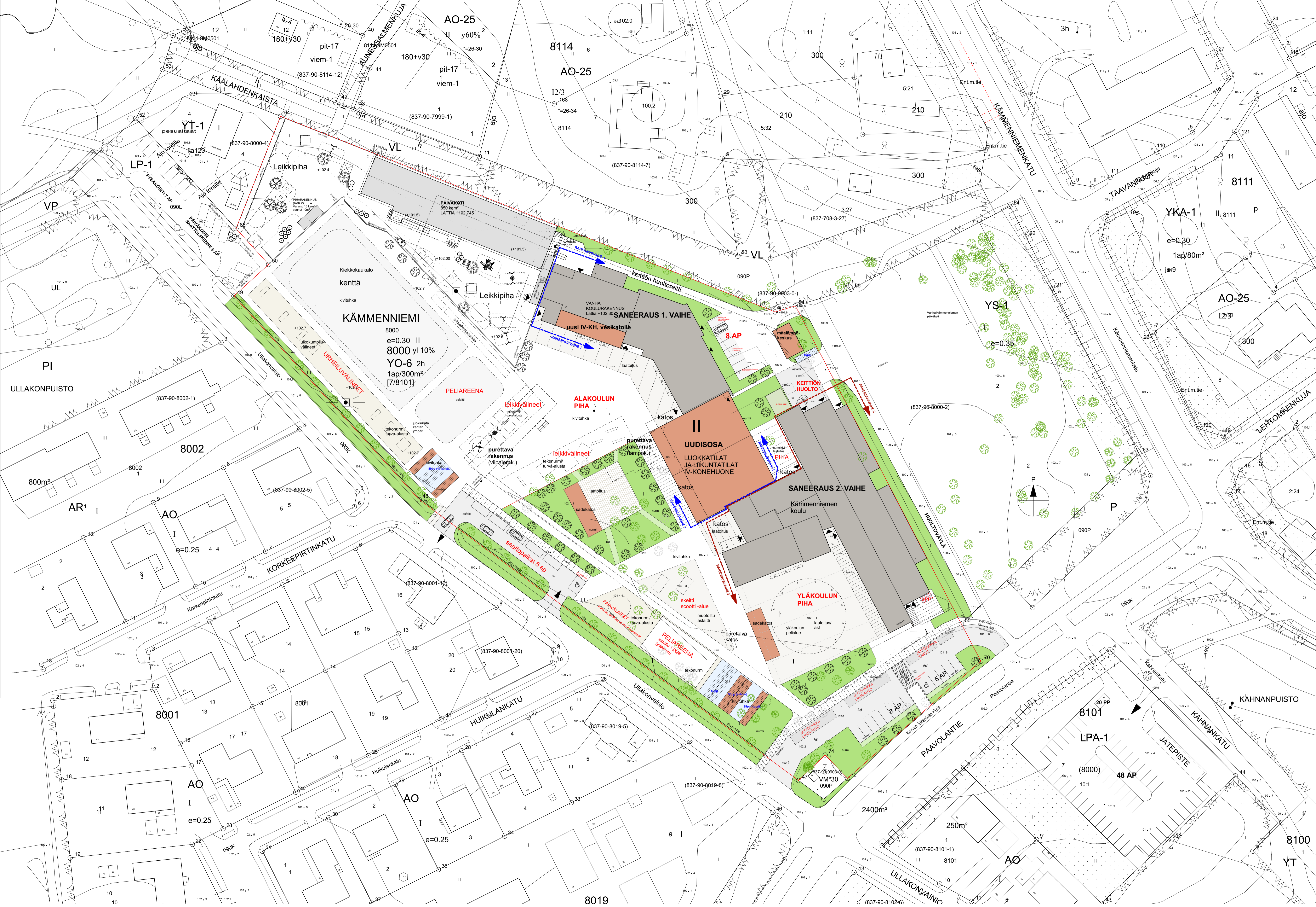
KÄMMENNIEMEN KOULU, Tarveselvitysluonnos VAIHTOEHTO -00 1:500 21.12.2023 Ark.tsto Tilatakomo Oy.
